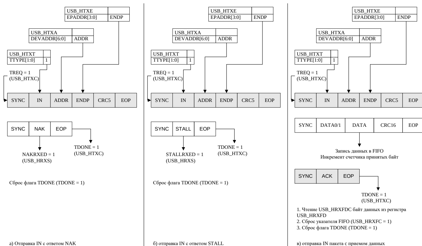
Рисунок 35 – Транзакция IN (USB Host)
