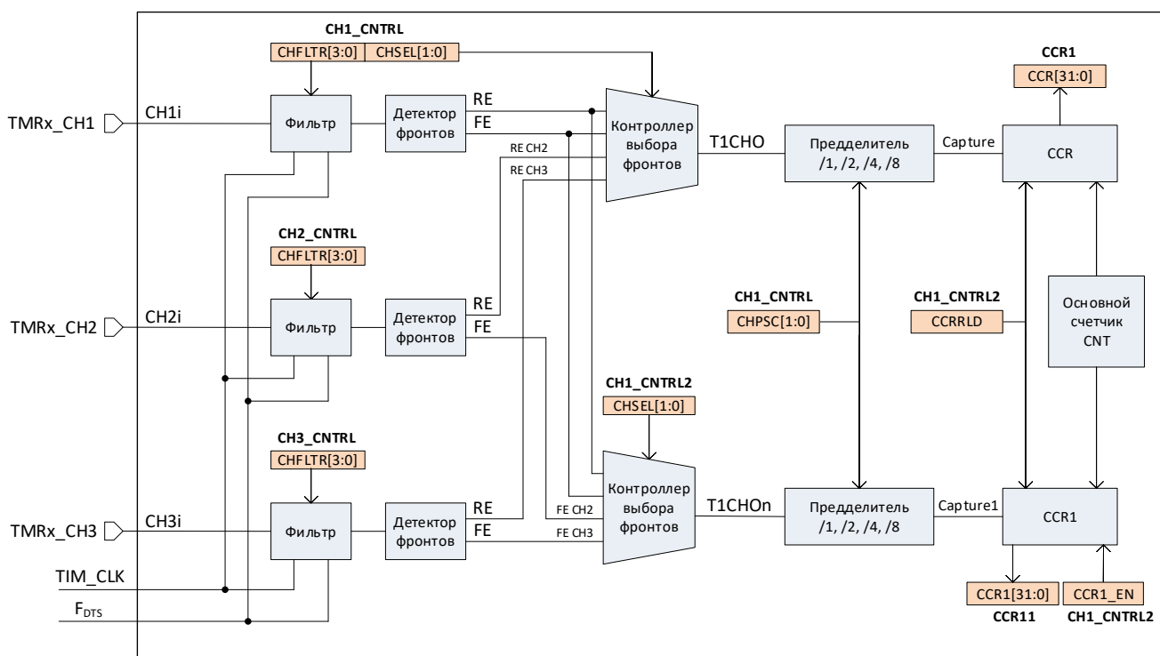
Рисунок 77 – Структурная схема блока захвата на примере канала 1
