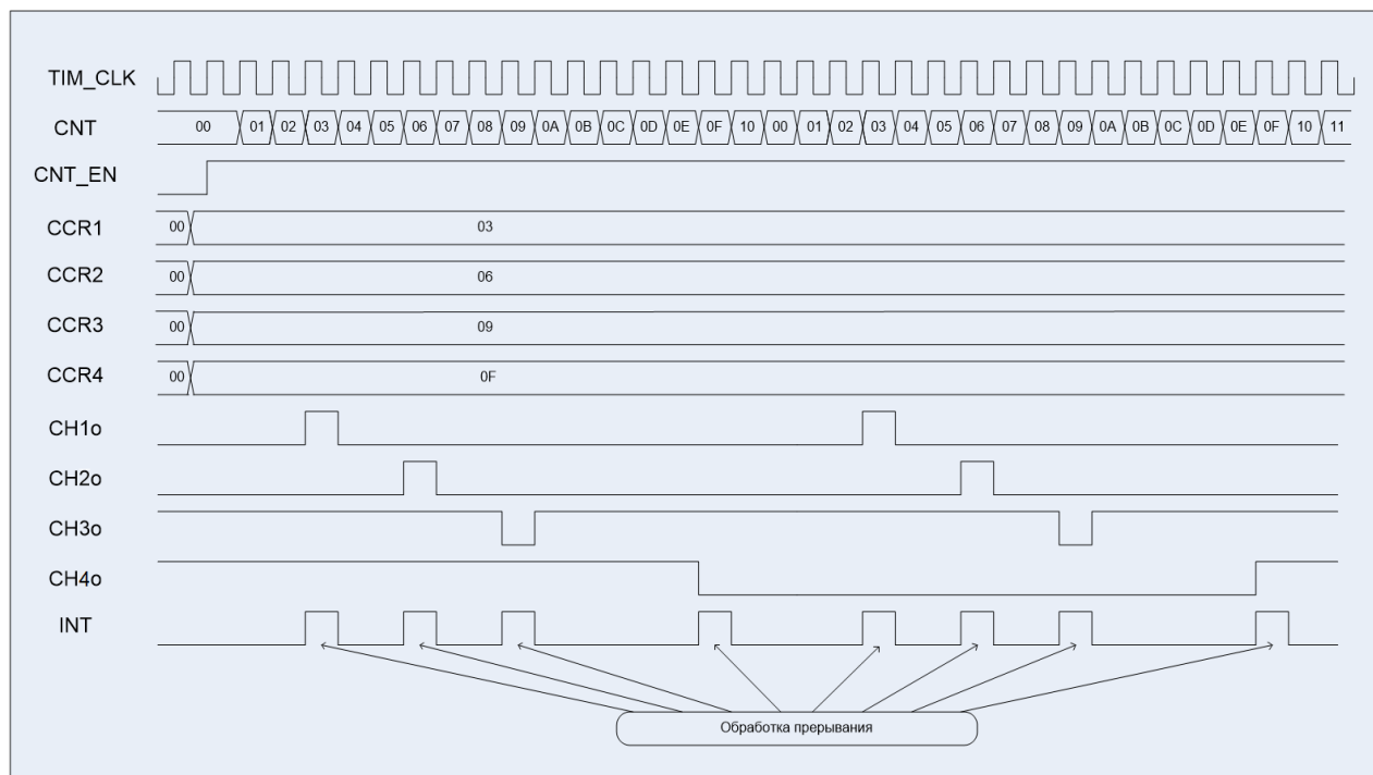
Рисунок 89 – Диаграммы примера работы в режиме ШИМ
