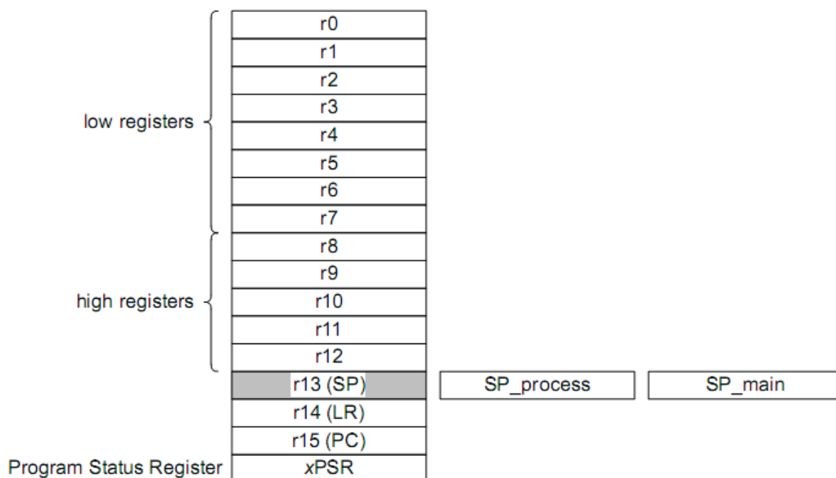
Рисунок 17 – Регистры ядра
