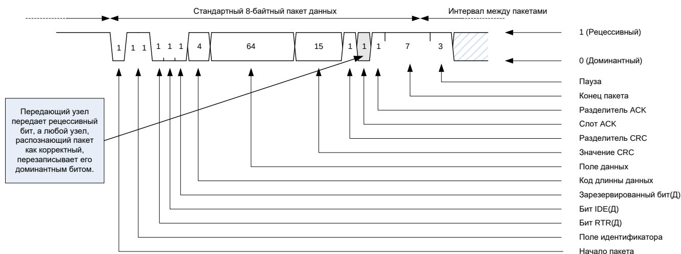
Рисунок 48 – Контроль подтверждения
