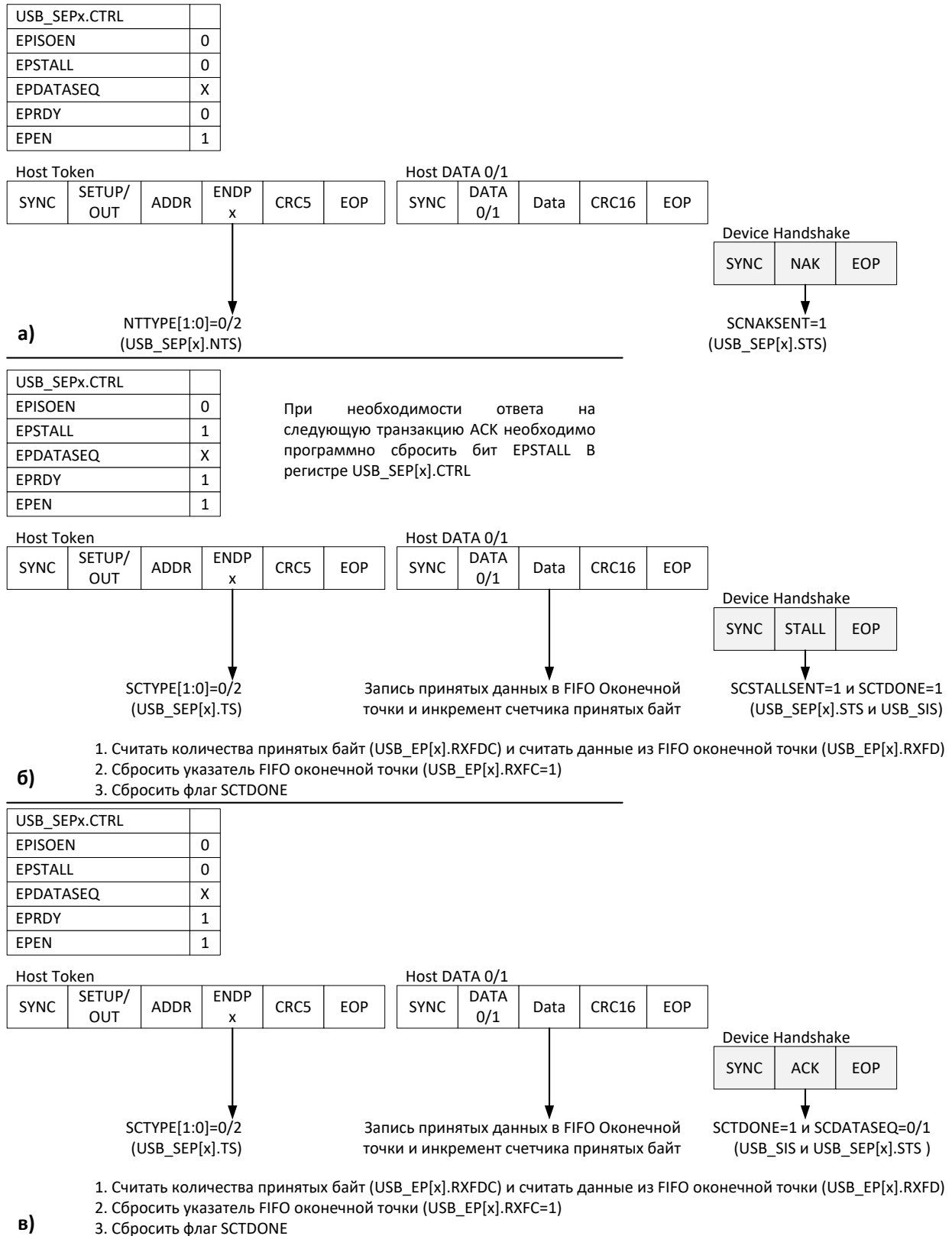
Рисунок 33 – Транзакция SETUP/OUT (USB Device)
