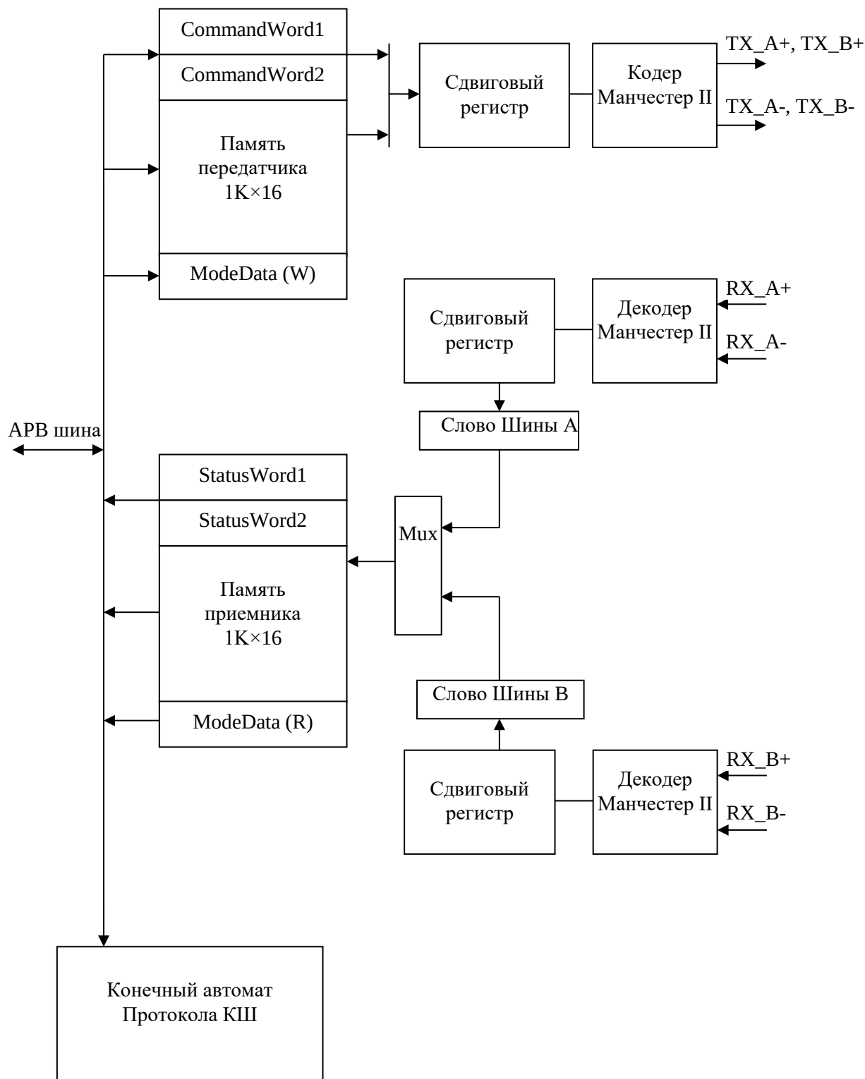
Рисунок 58 – Структурная схема работы в режиме КШ
