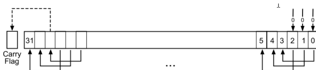
Рисунок 20 – Инструкция LSL # 3
