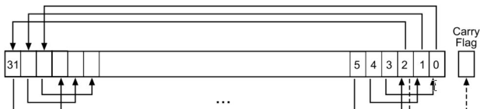
Рисунок 21 – Инструкция ROR # 3
