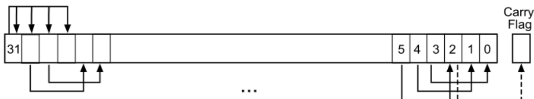
Рисунок 18 – Инструкция ASR # 3
