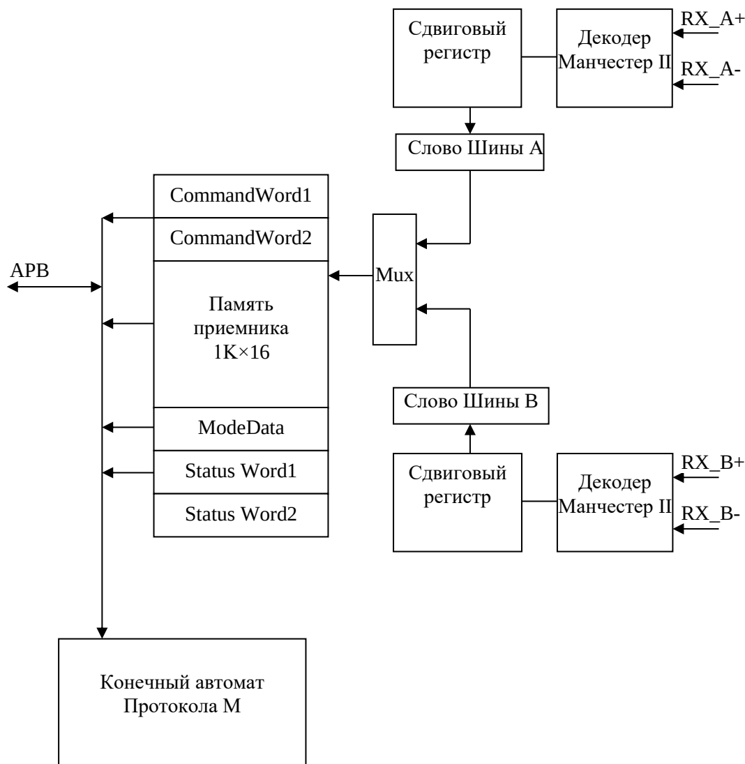
Рисунок 60 – Структурная схема работы в режиме М
