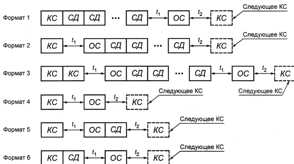
Рисунок 55 – Форматы сообщений
