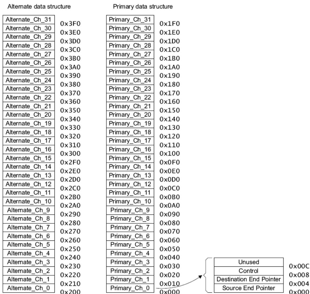
Рисунок 129 – Карта памяти для 32 каналов, включая альтернативную структуру управляющих данных
