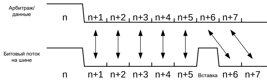
Рисунок 51 – Битстаффинг
