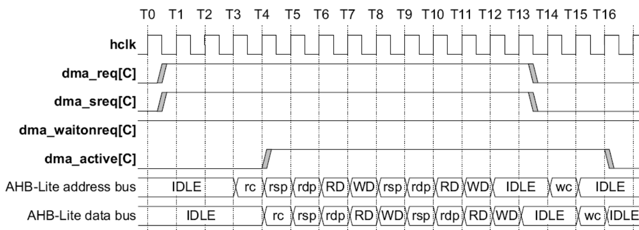
Рисунок 123 – Диаграмма работы контроллера DMA при использовании dma_waitonreq
