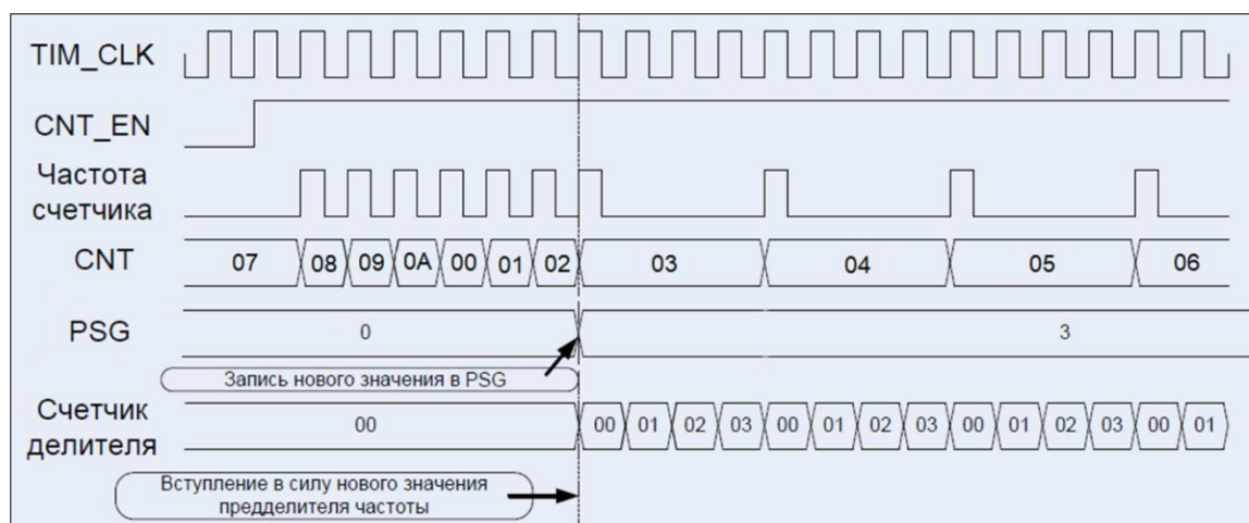
Рисунок 69 – Диаграмма работы счетчика: счет прямой (CNT_MODE[1:0] = 00, EVENT_SEL[3:0] = 0000, DIR = 0)
