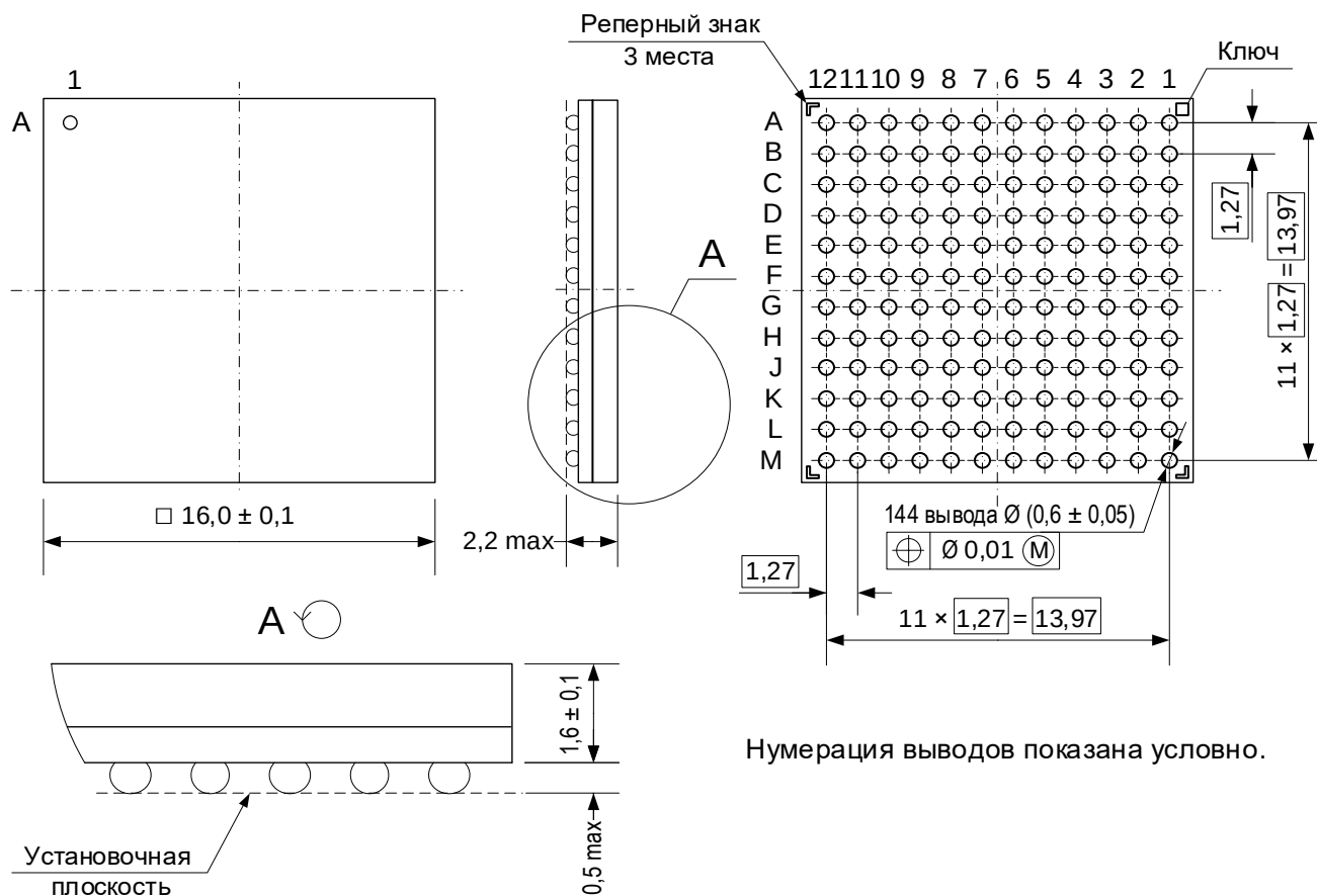
Рисунок 146 – Габаритный чертеж микросхемы K1986BE1GI в корпусе BGA144 16×16×1,6 (1,27)
