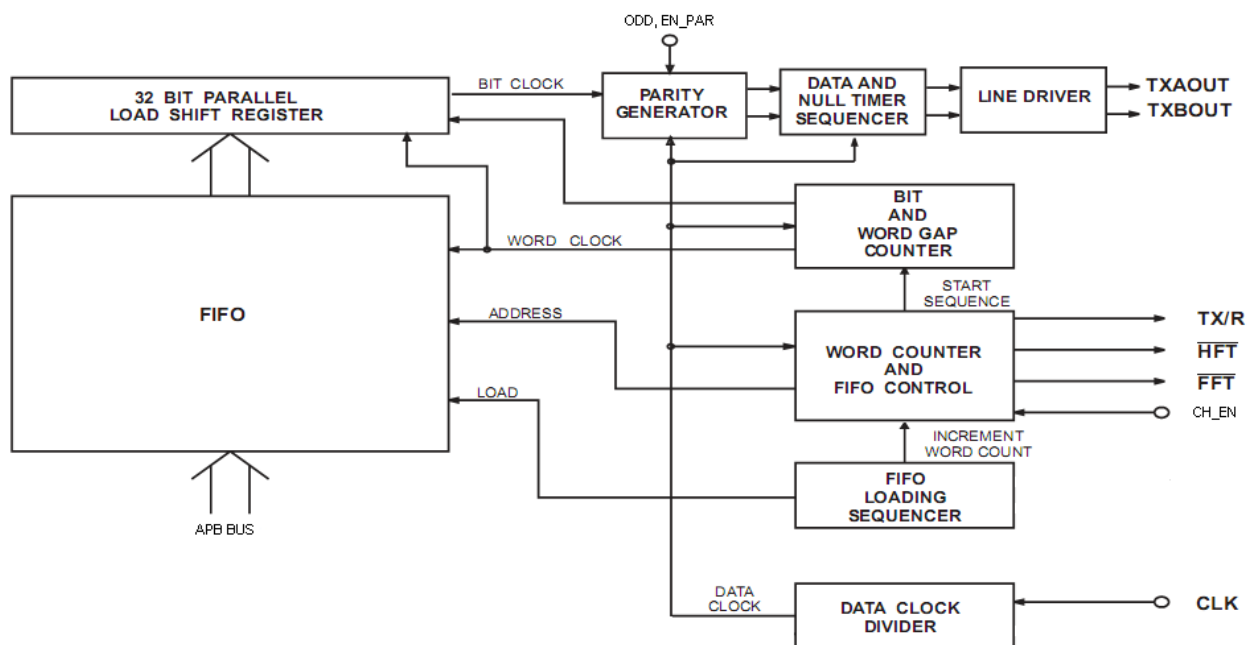
Рисунок 95 – Структурная схема канала передачи
