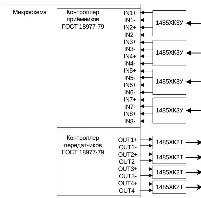
Рисунок 92 – Структура блока контроллера интерфейса по ГОСТ 18977-79
