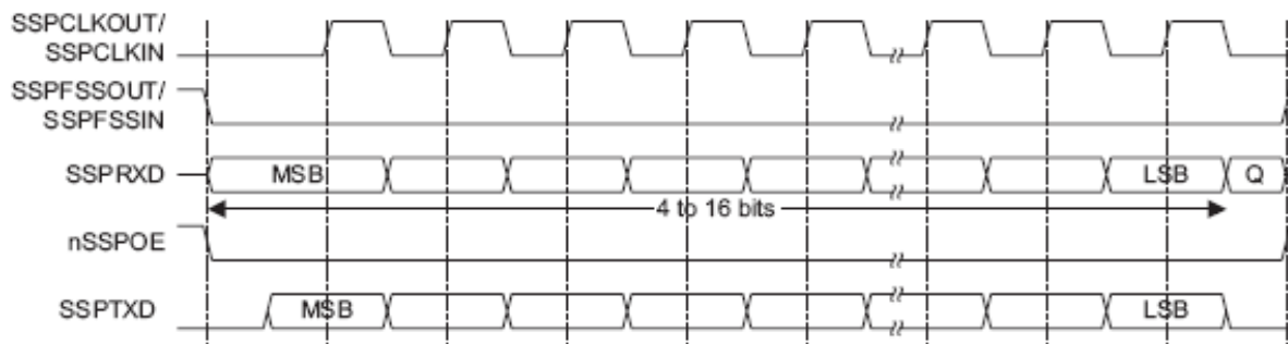
Рисунок 99 – Формат синхронного обмена протокола SPI, SPO=0, SPH=0 (одиначный обмен)
