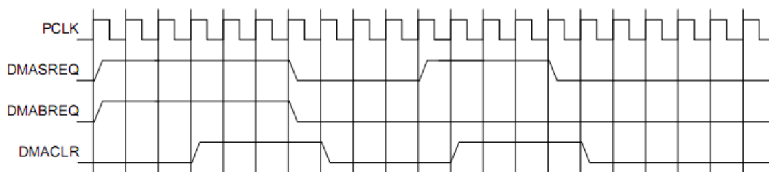
Рисунок 118 – Временные диаграммы одноэлементного и блочного запросов DMA
