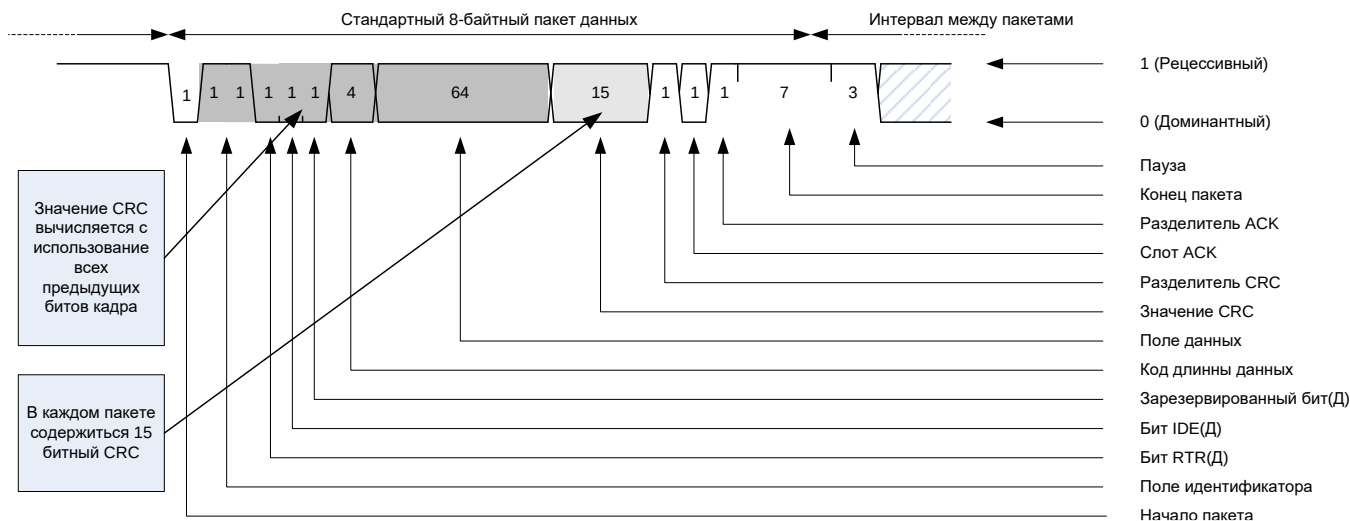
Рисунок 49 – Контроль CRC
