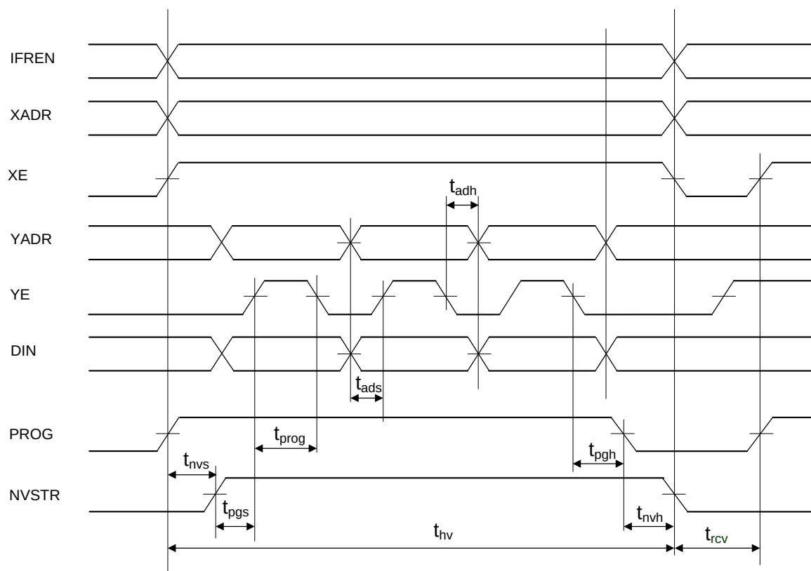
Рисунок 15 – Временная диаграмма чтения памяти
