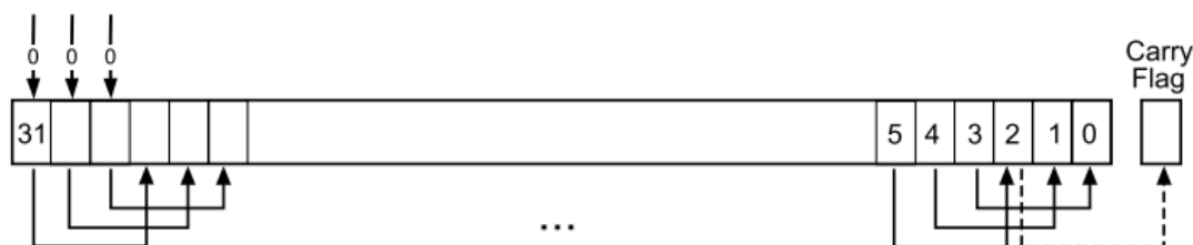
Рисунок 19 – Инструкция LSR # 3
