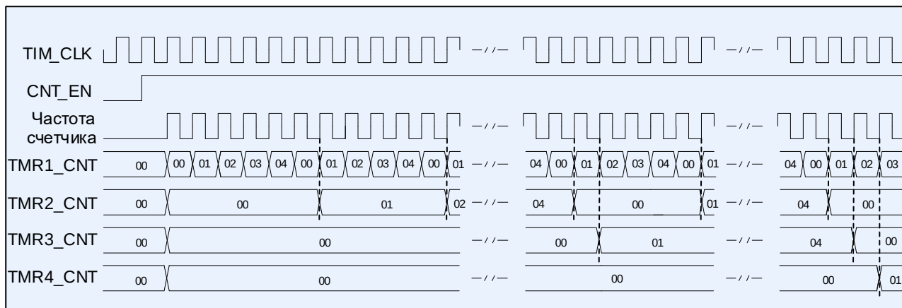
Рисунок 72 – Диаграммы работы четырех таймеров в каскаде TIMER1: DIR = 0, EVENT_SEL[3:0] = 0000, CNT_MODE[1:0] = 00; TIMER2: DIR = 0, EVENT_SEL[3:0] = 0001, CNT_MODE[1:0] = 10; TIMER3: DIR = 0, EVENT_SEL[3:0] = 0010, CNT_MODE[1:0] = 10; TIMER4: DIR = 0, EVENT_SEL[3:0] = 0011, CNT_MODE[1:0] = 10
