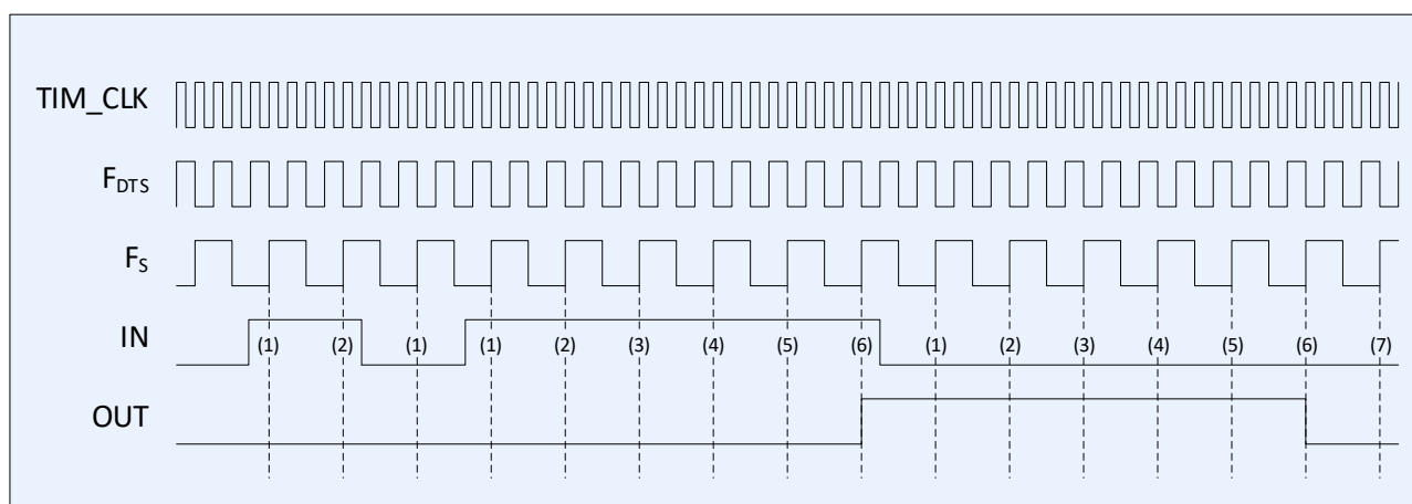
Рисунок 86 – Диаграмма работы фильтра, F_S = F_{DTS}/2 , N = 6
