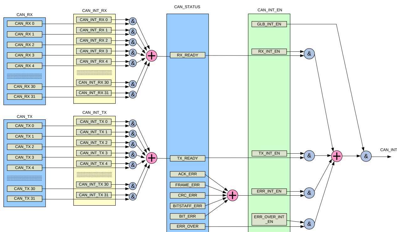
Рисунок 53 – Схема формирования прерывания блока CAN
